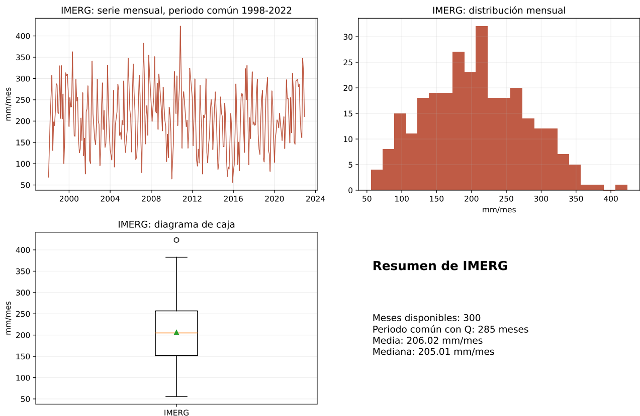
Figura 15: IMERG incorporado al análisis: serie cronológica, distribución, diagrama de caja y resumen del periodo común.
